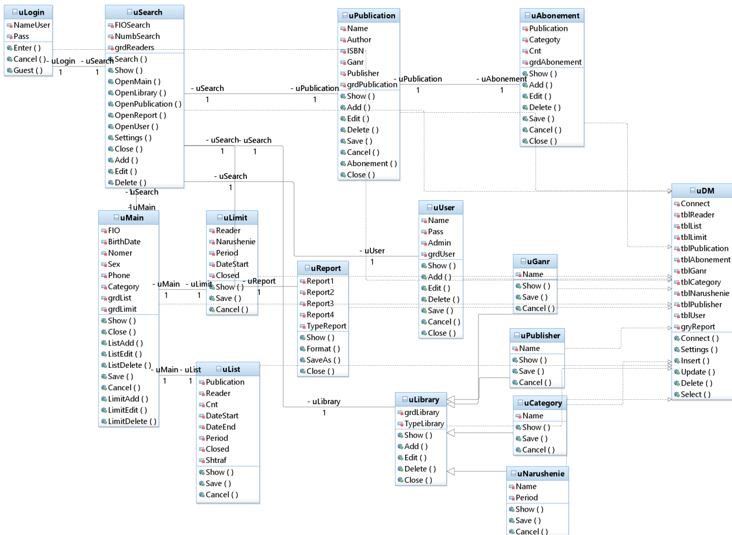
Рисунок 2.2 – Диаграмма классов
